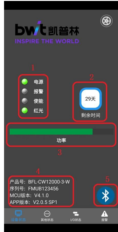
图 6 设备状态界面
